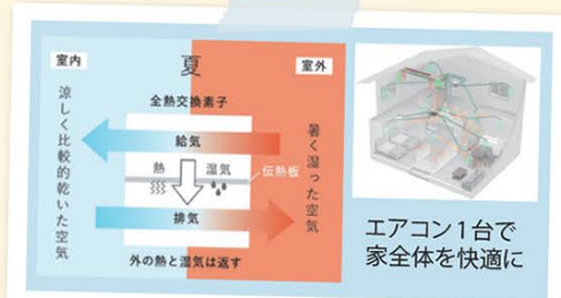
全館空調熱交換システム「ウイズエア」
